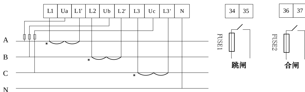
DTSY1352-NK 经互感器接入接线图
