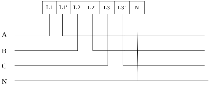
DTSY1352-NK 直接接入接线图
