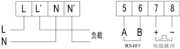
DDS1352-NK 接线图
