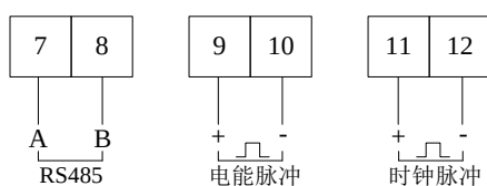
DTSY1352-NK 经互感器接入接线图
